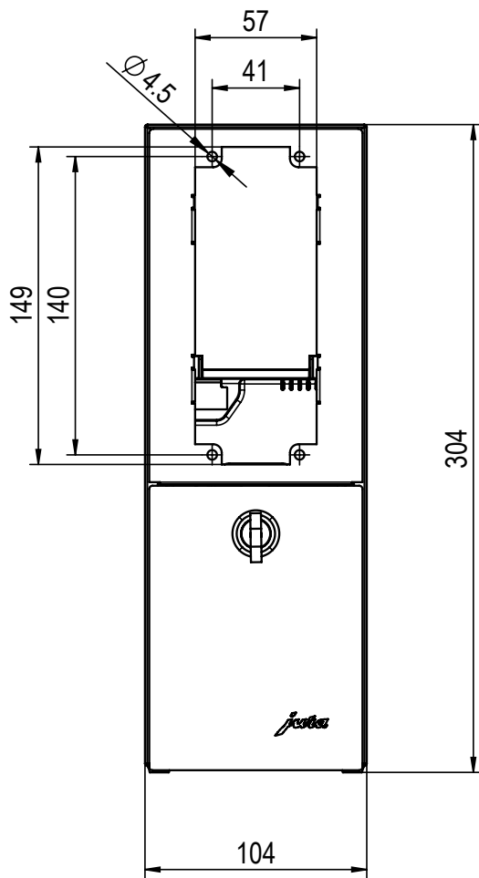
Aufriss
